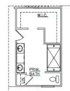
OPT 7ET SHOWER
